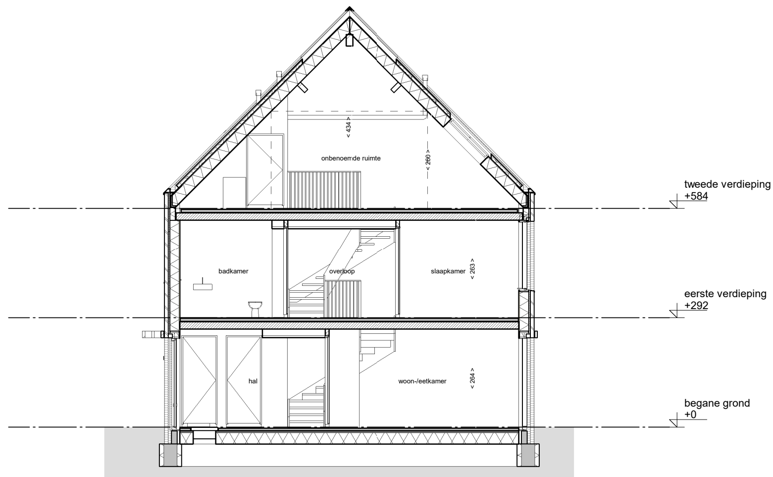
doorsnede
